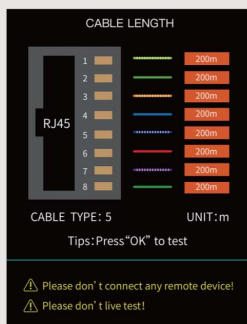
RJ-45 길이측정
